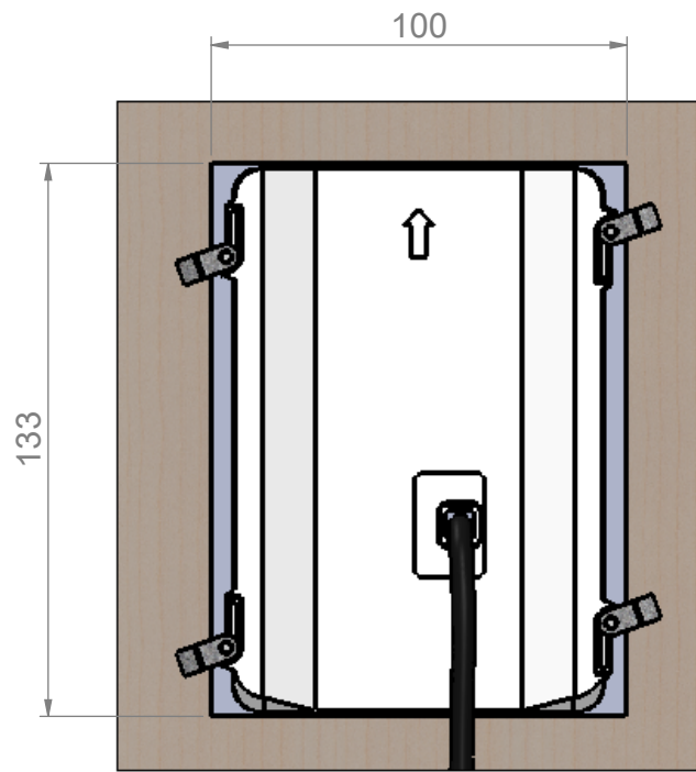
Cutout Dimensions
