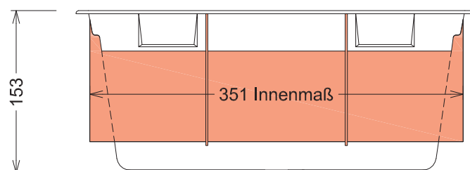
Ansicht Skimmerseite
