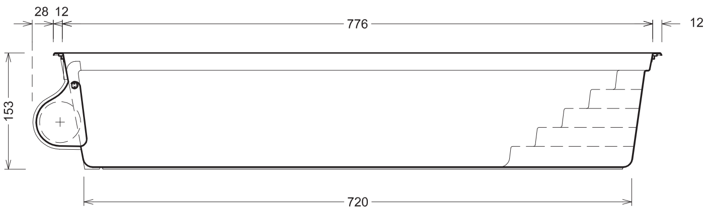
Schnitt
