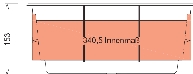
Ansicht Skimmerseite
