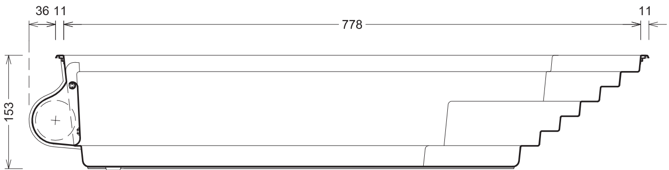
Schnitt
