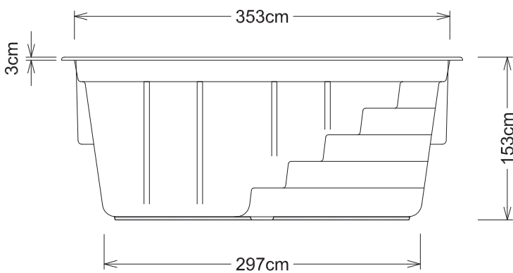
Ansicht Treppenseite
