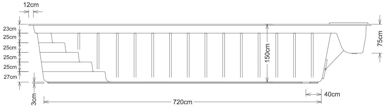
Seitenansicht
