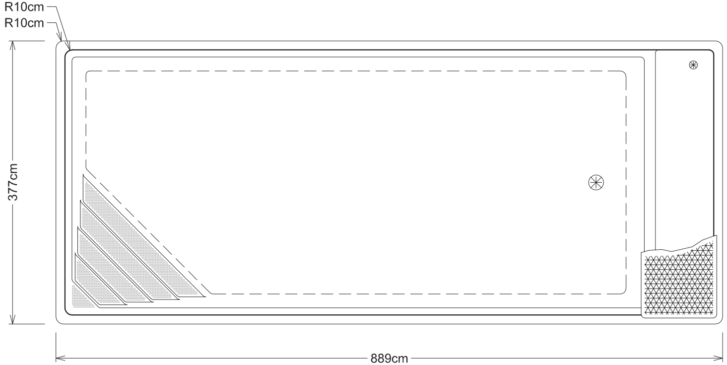
Grundriss
