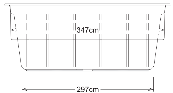
Ansicht Skimmerseite
