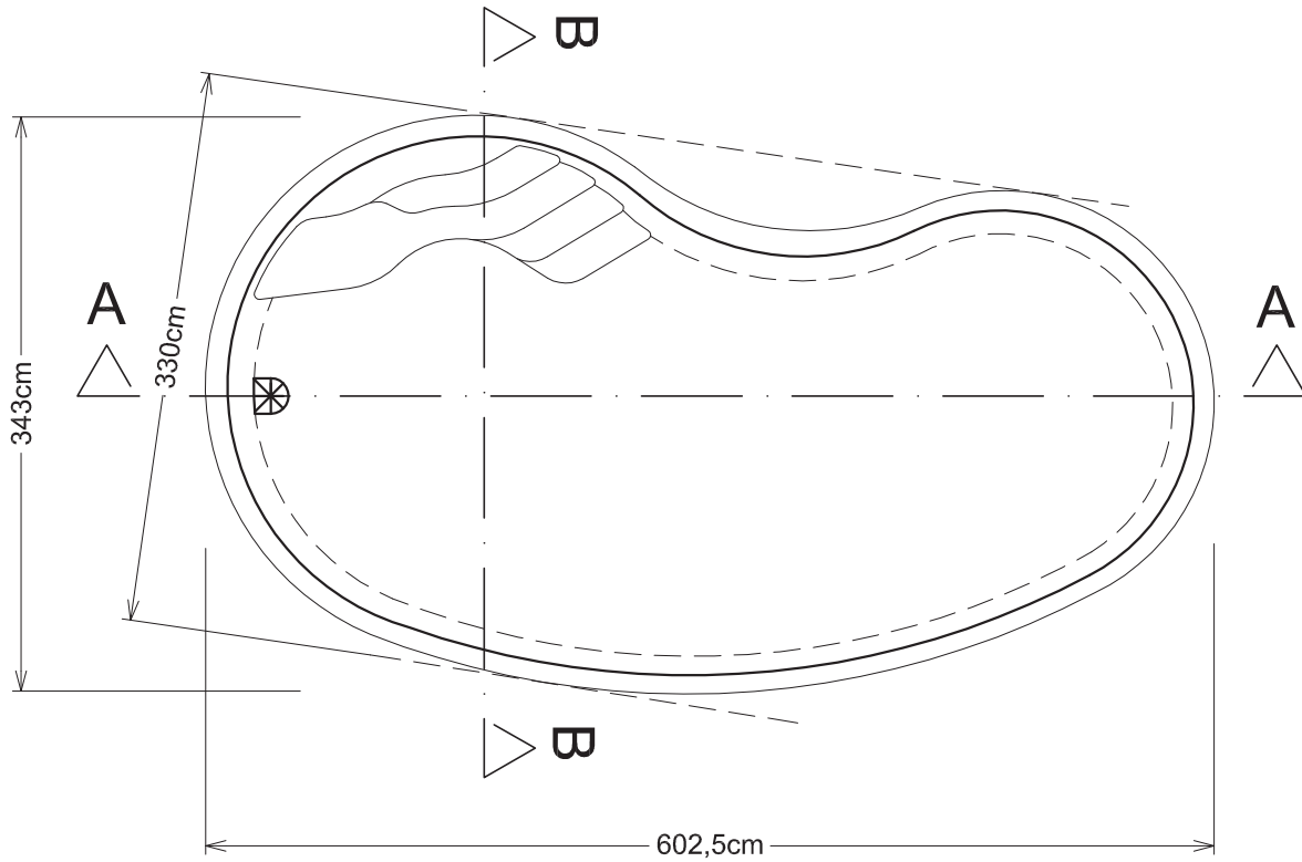
Grundriss
