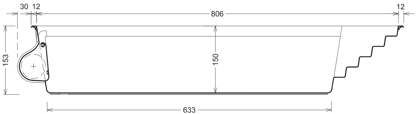
Schnitt
