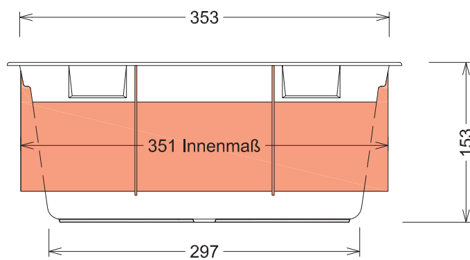
Ansicht Skimmerseite
