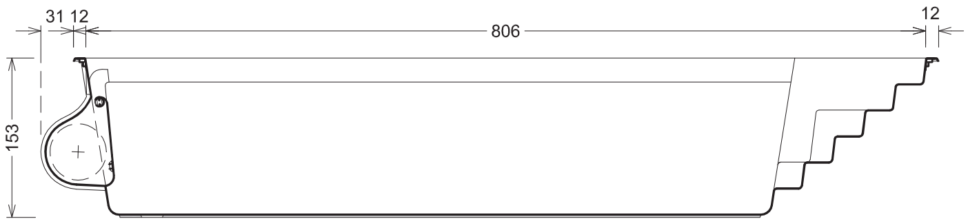
Schnitt
