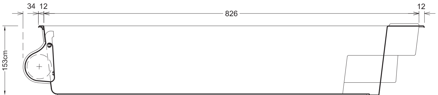
Schnitt
