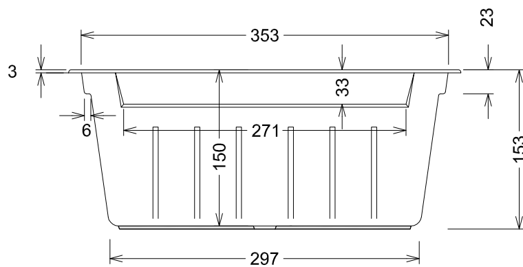
Ansicht Skimmerseite
