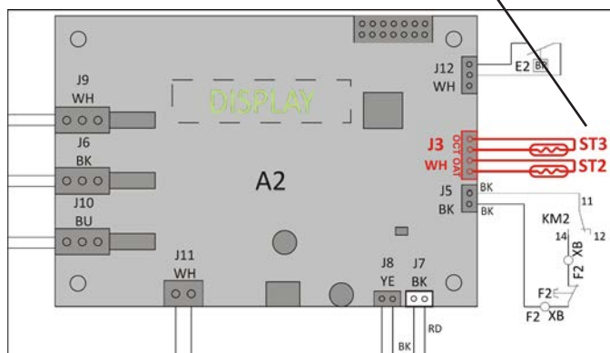
ST3 Abtaufühler
