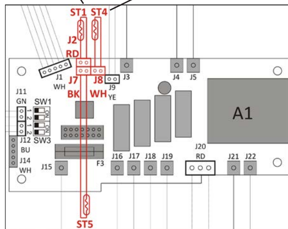
ST5 Fühler an der Druckseite des Kompressors
